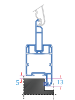
TELAIO SU TRE LATI E ANTA SOTTO IN BATTUTA
